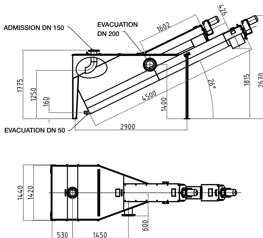
Schéma standard DA 320
